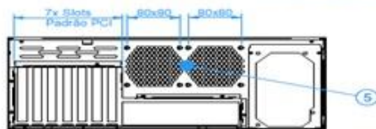
Painel traseiro SEÇÃO A-A
